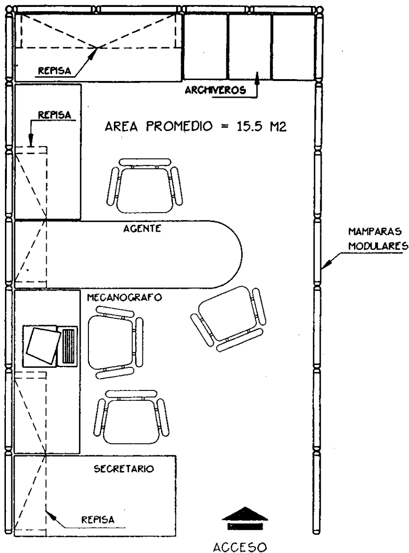
MODULO TIPO AGENTE MINISTERIO PUBLICO ESPECIALIZADO
