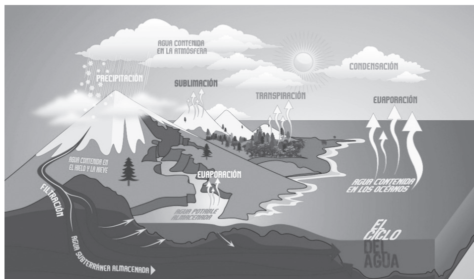
Figura 1. Ciclo hidrológico
